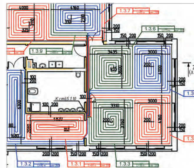
Детский сад. Уфа (Башкортостан) Фрагмент проекта водяного напольного отопления
