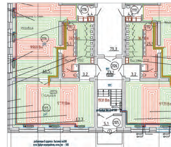
Школа. Тобольск (Тюменская область) Фрагмент проекта водяного напольного отопления
