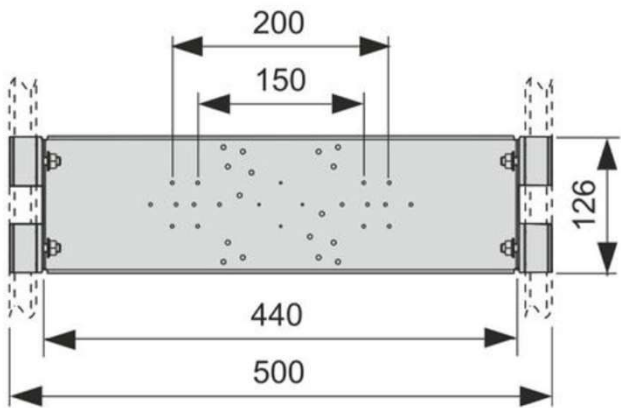
Основные установочные размеры
