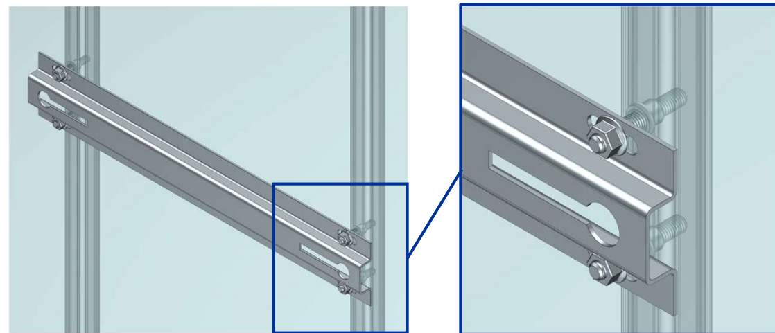
Применение резьбовых заклепок М8 для установки монтажной планки
