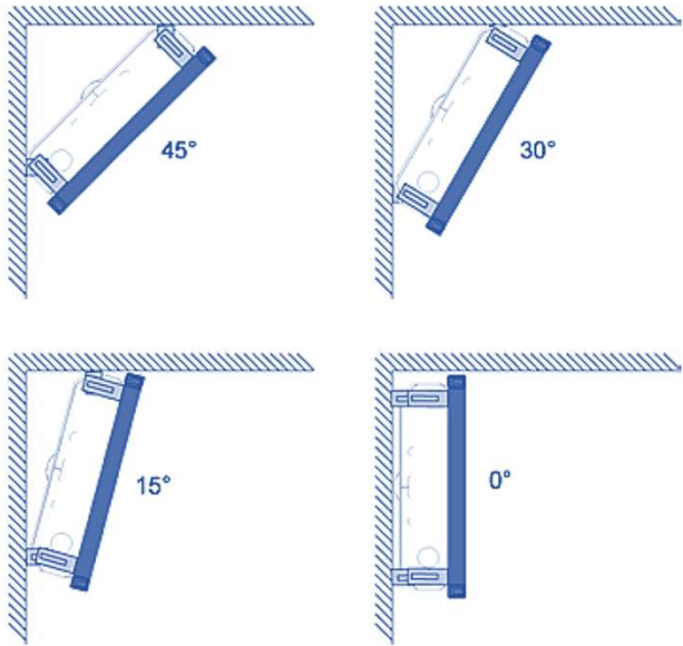
Пример установки инсталляции под различным углом
