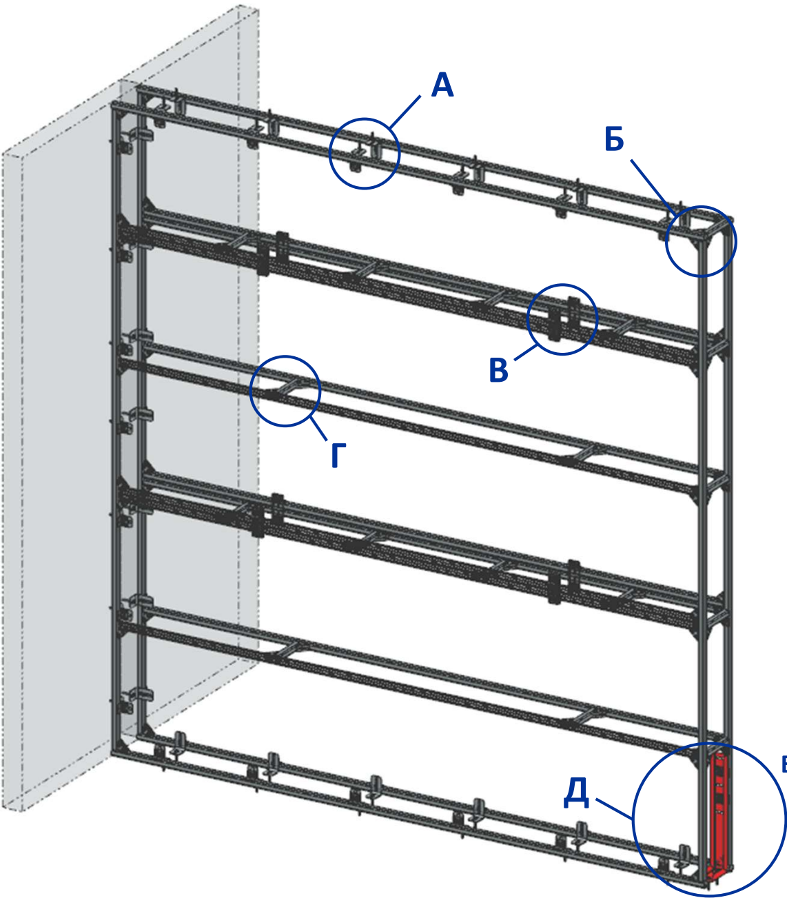
В – Крепление универсальное WB90182 Г – Ребро жесткости WB90003 + 2x WB90102
