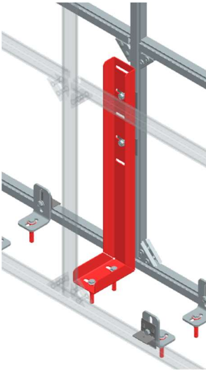
Д – Опора для отдельной перегородки WB90317
