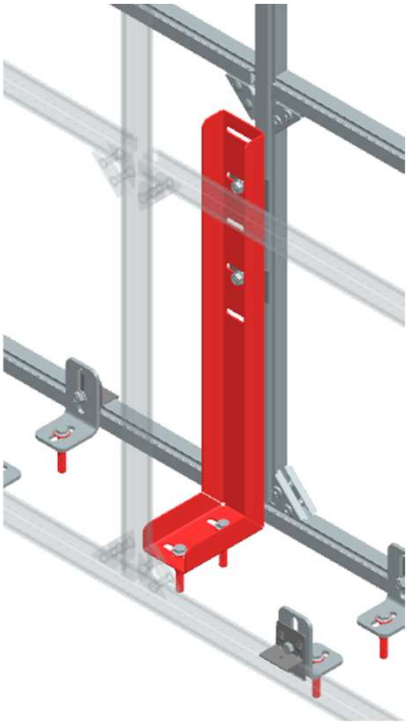
Д – Опора для отдельностоящей перегородки WB90317
