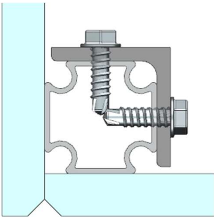
Прилегание листов обшивки с внешнего угла конструкции
