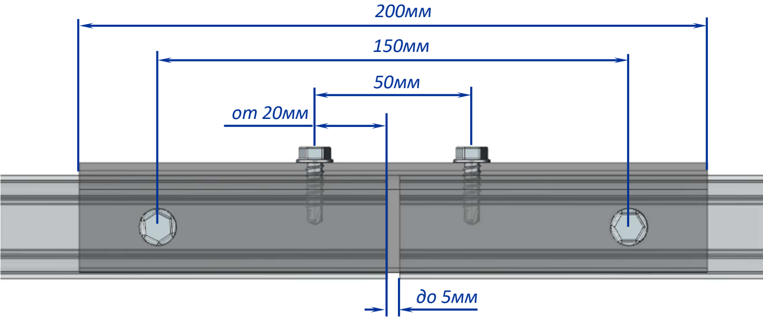
Установочные размеры уголка для наращивания профиля WB90109
