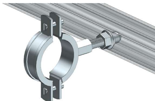
Применение резьбовой заклепки М8 для установки трубного хомута
