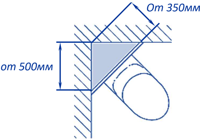
Минимальные размеры под установку инсталляции в углу
