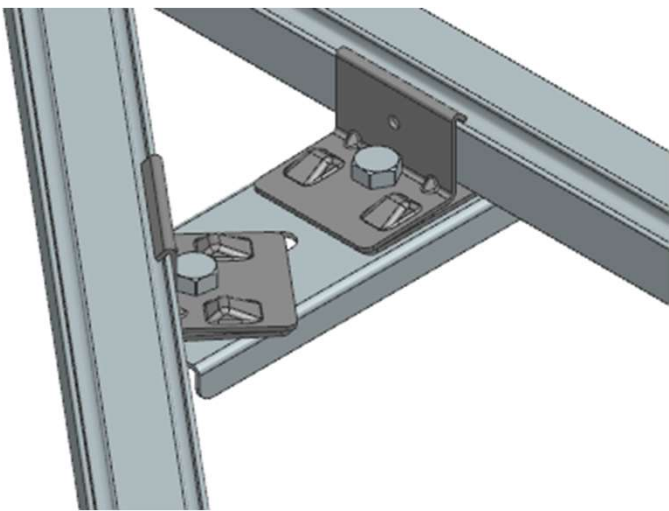
Соединение под углом
