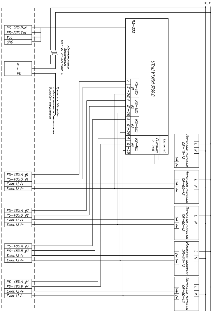
Рисунок 1 – Структурная схема щита автоматизации VT.WM.700.19
