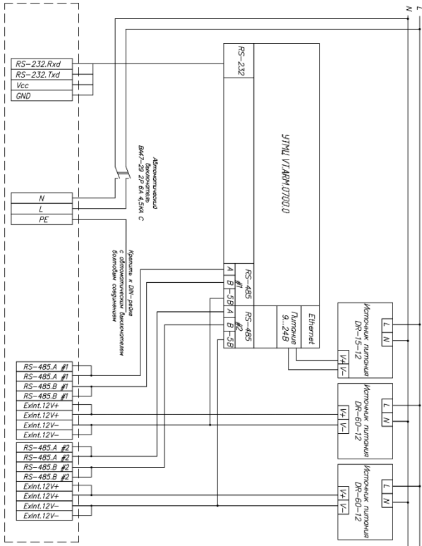
Рисунок 2 – Структурная схема щита автоматизации VT.WM.700.20
