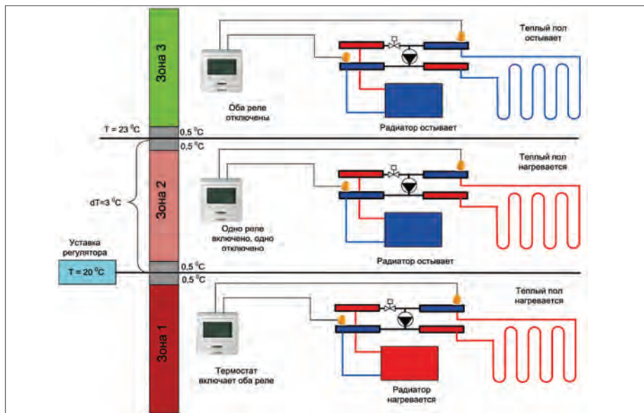
Рис. 29. Двухконтурное управление комбинированной системой отопления
