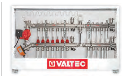
Комбинируемая система на базе узла VT.DUAL
