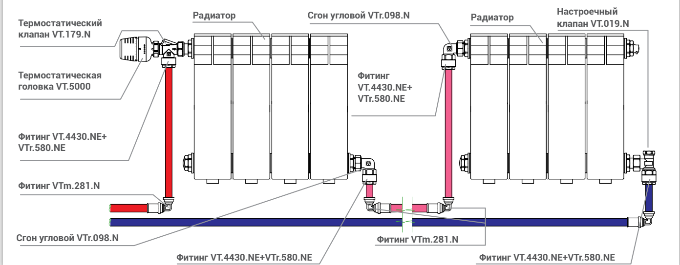
Рис. 24 Последовательное подключение приборов при комбинированной схеме
