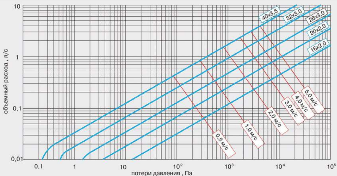
Номограмма определения потерь давления в металлополимерных трубах
