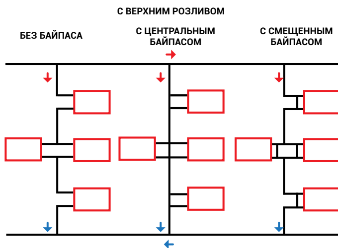
Рис. 1 Однотрубные вертикальные системы
