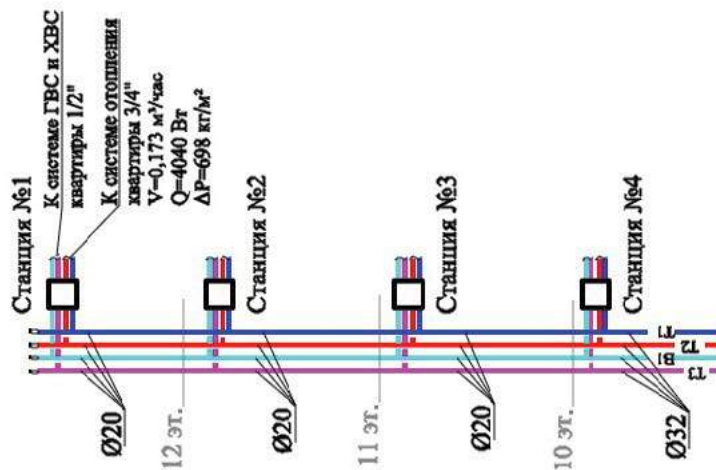
Схема типового стояка Т1, Т2, В1, Т3
