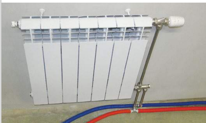
Рис. 8 Пример подключения радиатора с помощью фитинга VTm.282
