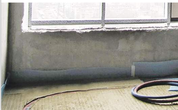
Рис. 6 Прокладка трубопроводов в штробах шумоизоляционных плит
