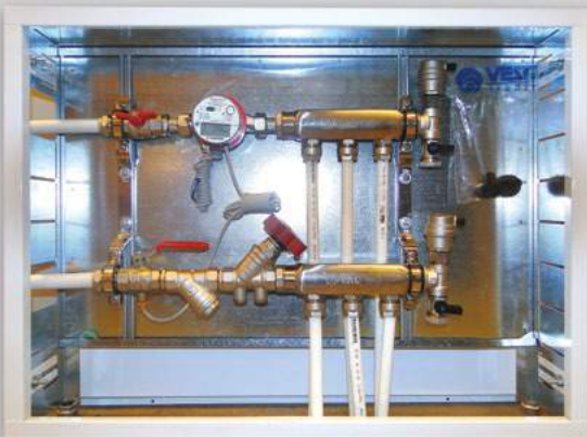
Рис. 21 Коллекторный шкаф с узлом учета тепловой энергии
