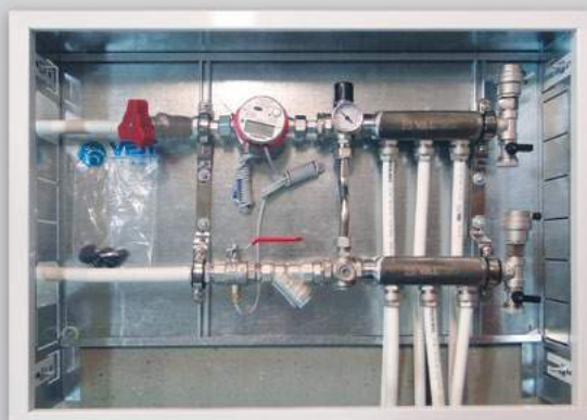
Рис. 22 Коллекторный шкаф с узлом учета и перепускным клапаном
