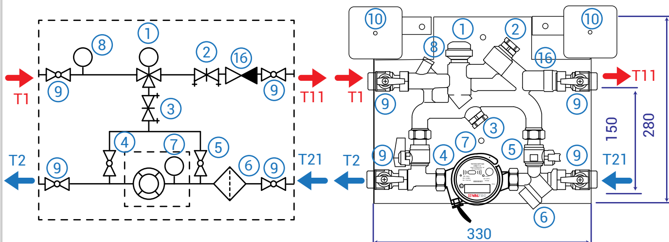
Рис. 13 Схема станции VALTEC Control Modul
