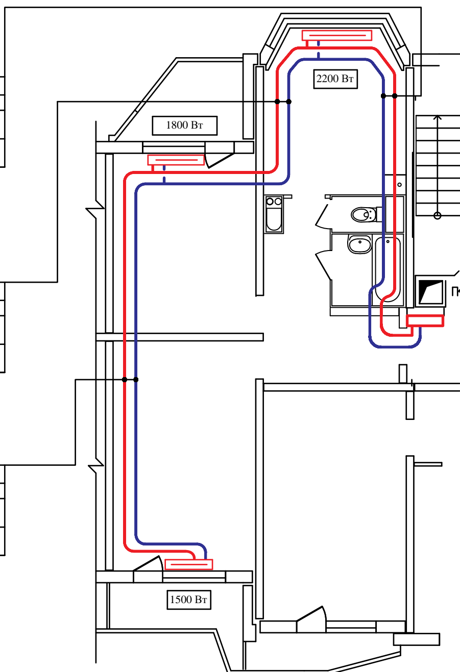
Расчетная схема
