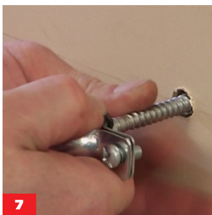
7 Устанавливаются неподвижные опоры
