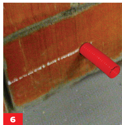
6 Устанавливаются гильзы из гофрированной трубы в отверстия стен и перегородок так, чтобы гильза выступала не менее чем на 50 мм за грань конструкции
