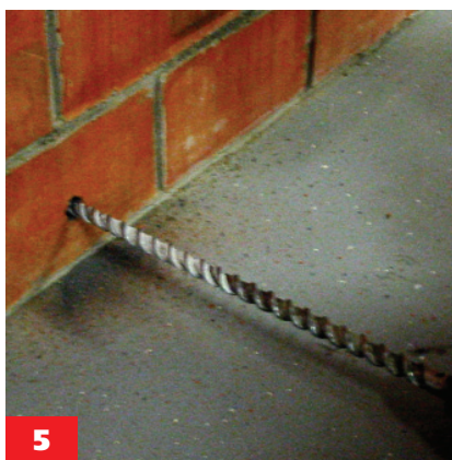
5 Пробиваются или высверливаются отверстия для прохождения трубы через стены и перегородки
